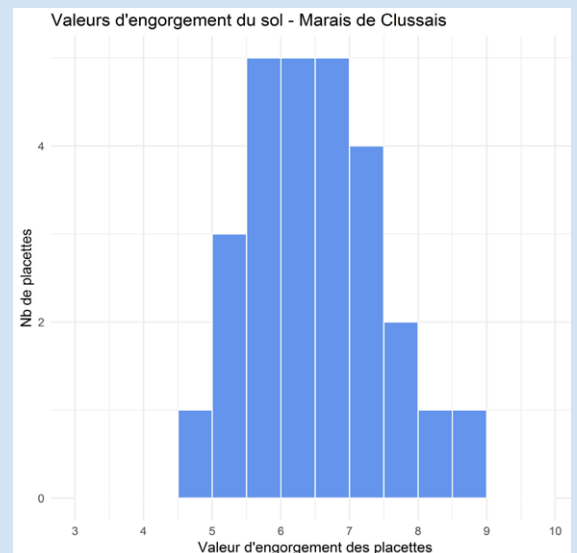
Figure 2 : valeur diagnostique de niveau d'engorgement des placettes de type SDAGE 10 en 2017
